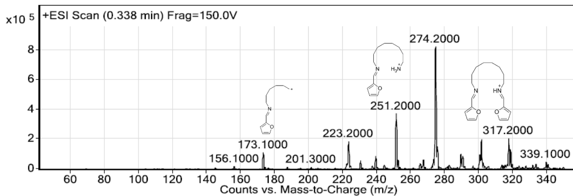
L 14 e ait LC- ESI/MS spektrumu
